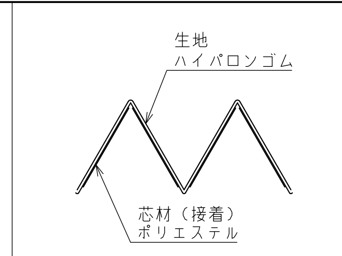
ジャバラ詳細図
