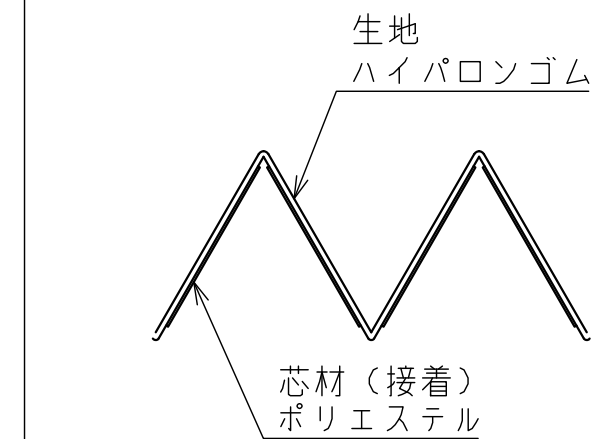
ジャバラ詳細図
