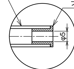
A部詳細
