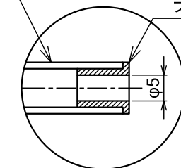
A部詳細
