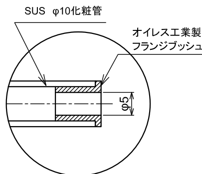
A部詳細
