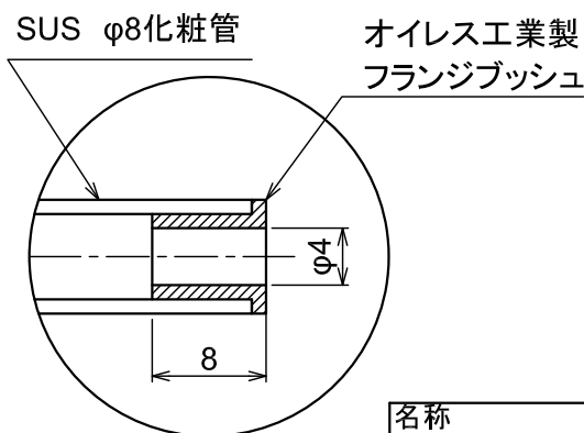
A部詳細
